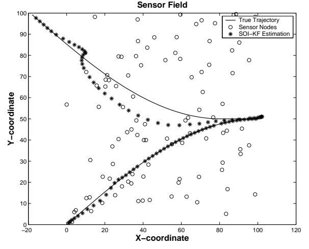
Fig. 2. SOI-KF estimation
