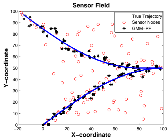
Fig. 4. GMM-PF estimation
